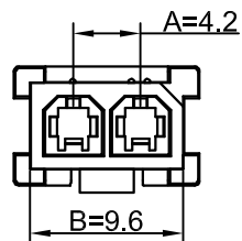
KB971-02H3A-XX 双孔防呆(旧模)
