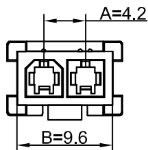
KB971-02H3B-XX 单孔防呆(新模)
